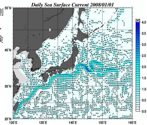
日本周辺の海流図 (気象庁 HP より)
