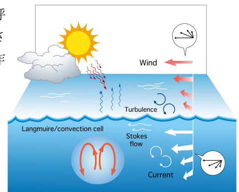
大気海洋境界層の模式図。
